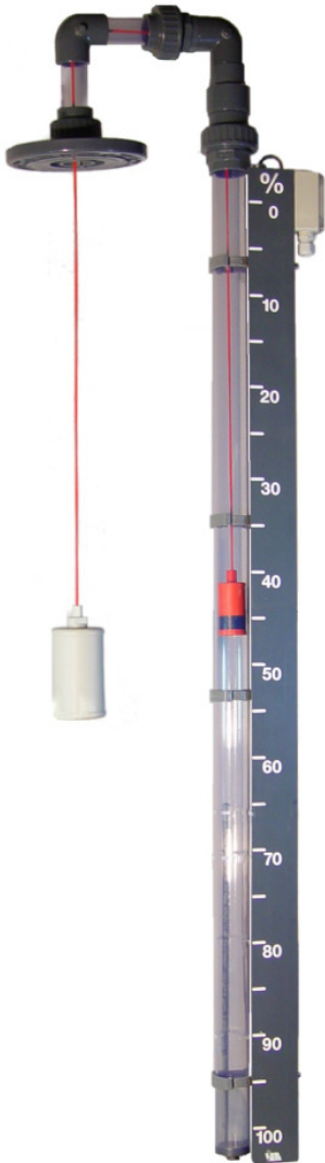
Seilzug-Füllstandanzeige *)
