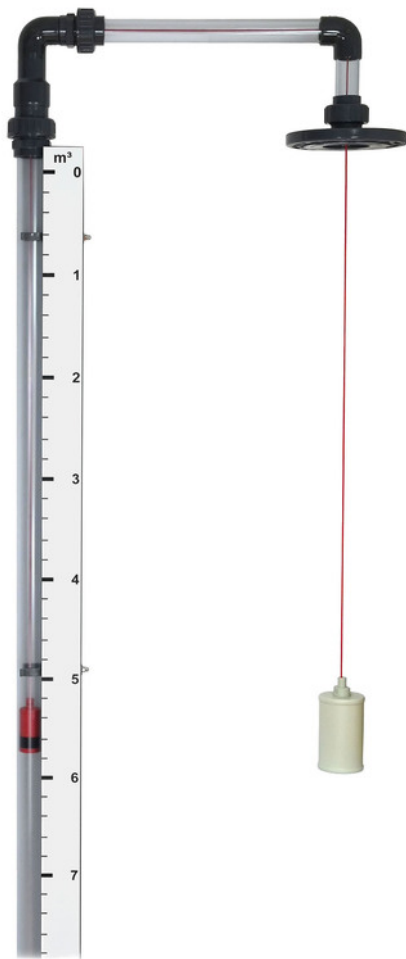
Seilzug-Füllstandanzeige *)
