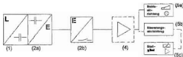
Leckagesonde mit externem Messumformer (2b)
