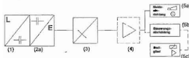
Leckagesonde mit integrierten Messumformern (2a) mit Strom-Ausgang
